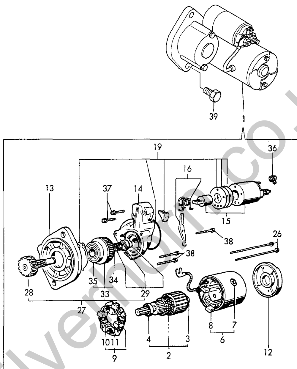
Fig. 16 スターティングモータ STARTING MOTOR
