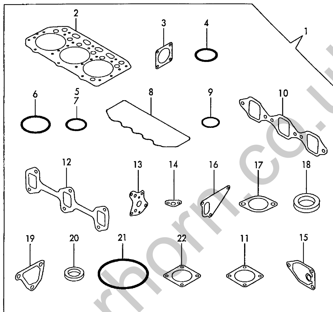
Fig. 18 バッキンセット (オプション) & 工具 GASKET SET (OPTIONAL) & TOOL
