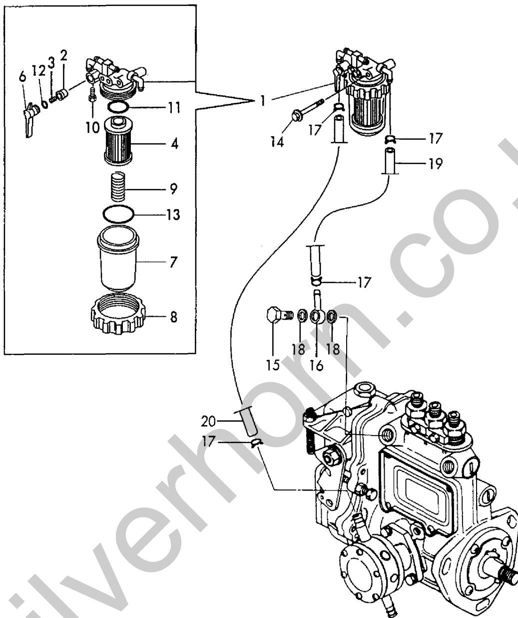
Fig. 14 燃料パイプ FUEL PIPE
