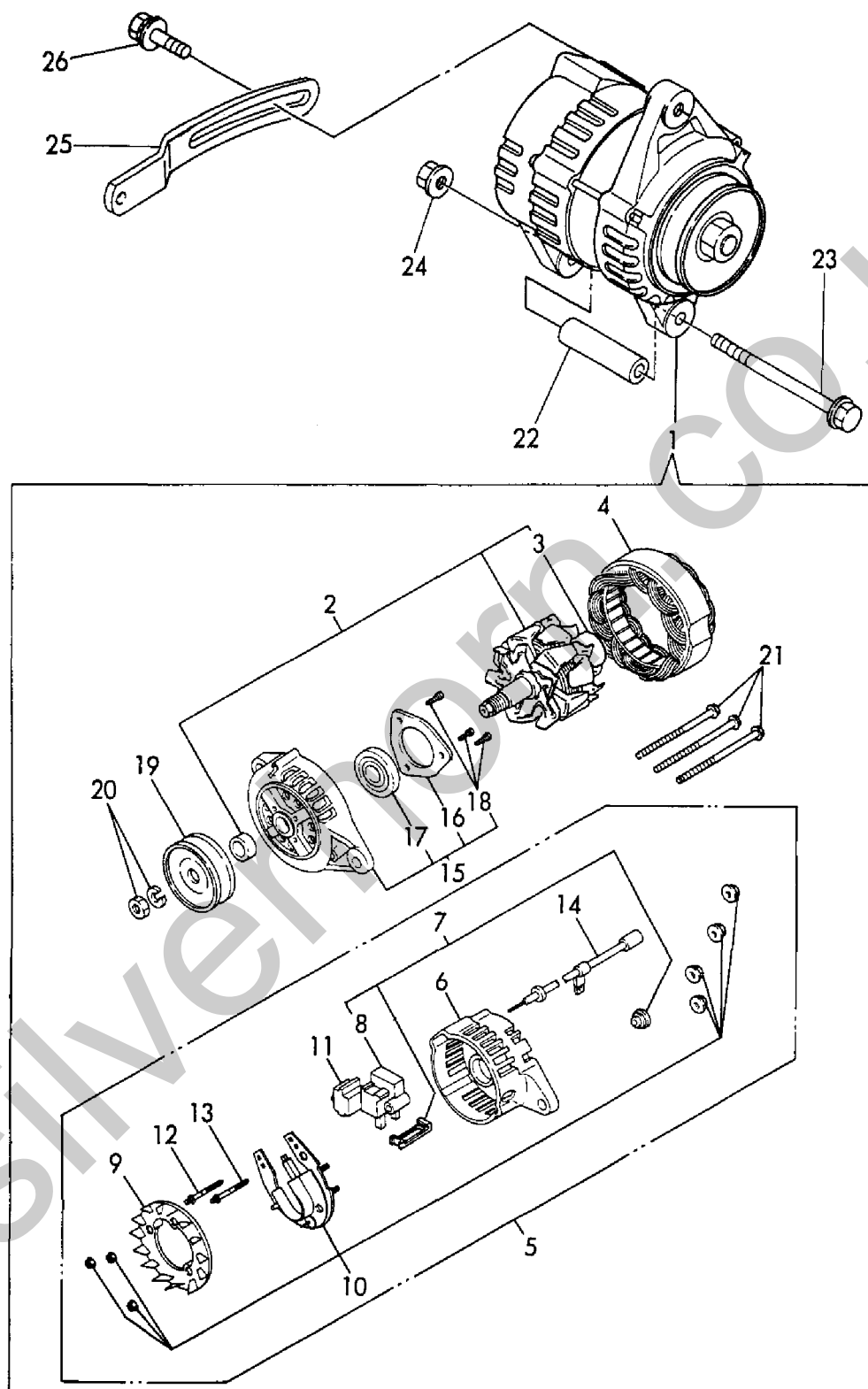
Fig. 17 ジェネレータ GENERATOR
