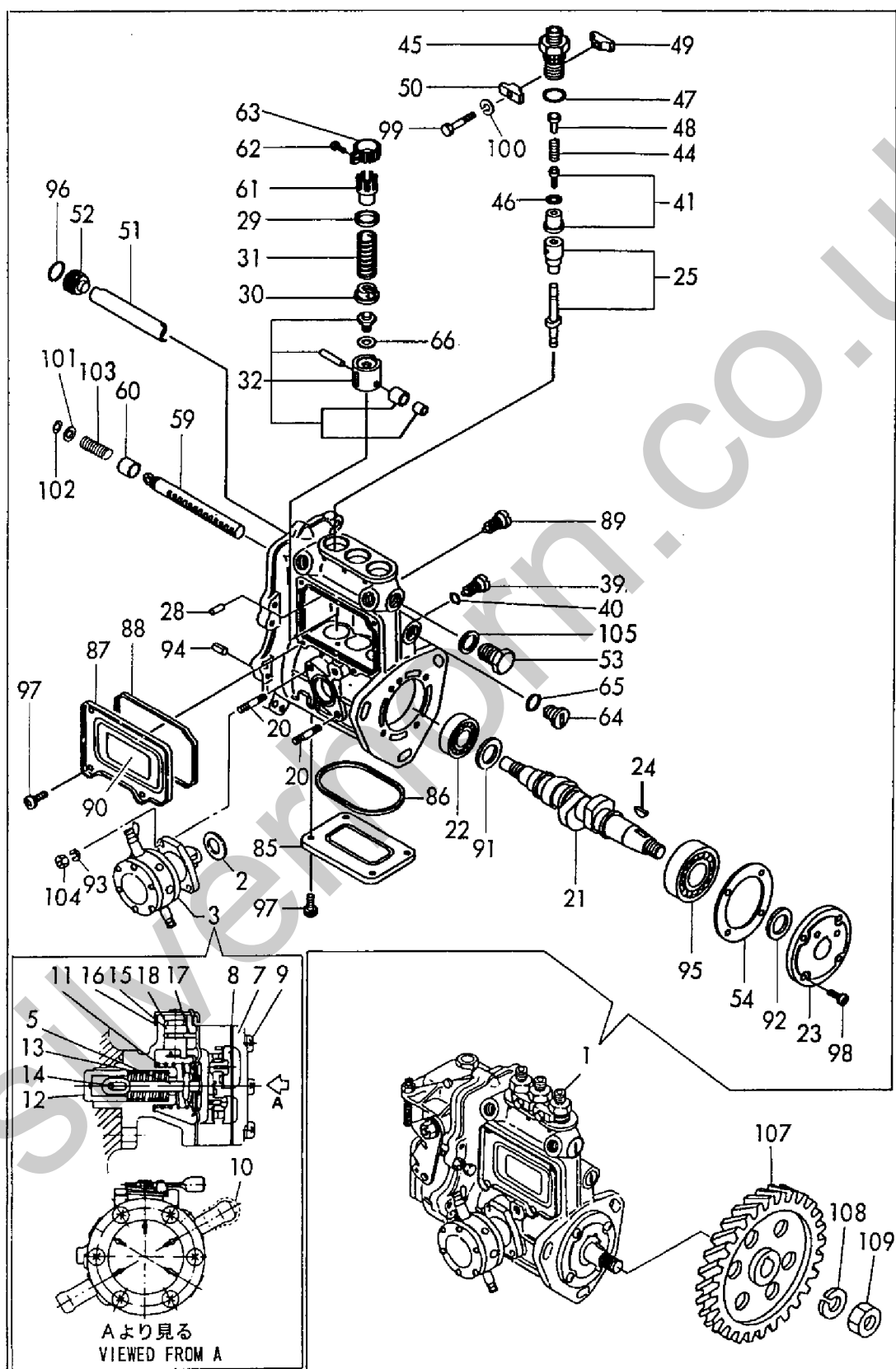
Fig. 11 燃料噴射ポンプ FUEL INJECTION PUMP
