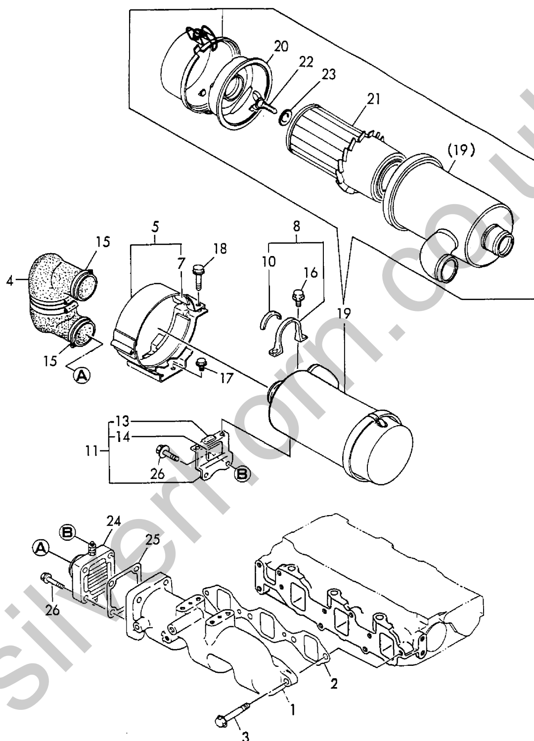
Fig. 5 吸気マニホールド&エアクリーナ SUCTION MANIFOLD & AIR CLEANER
