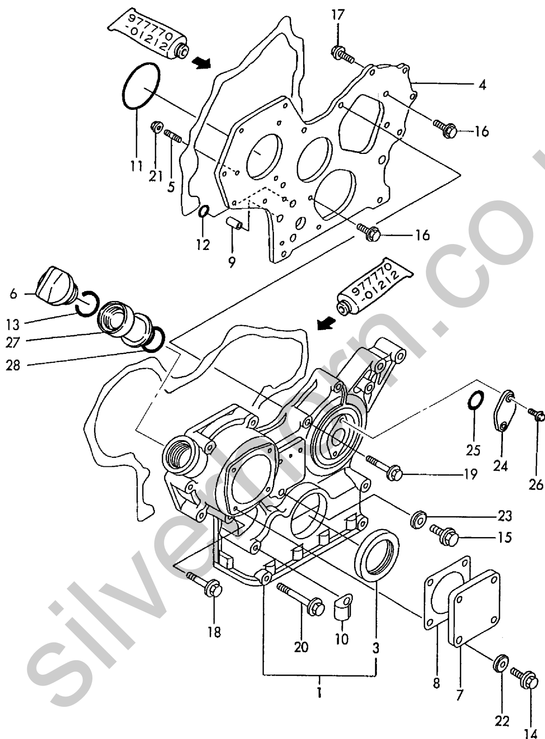
Fig. 2 ギヤケース GEAR HOUSING
